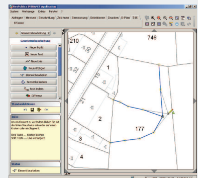
Abb: Topologisches Erfassen und Editieren von Geometrien.
